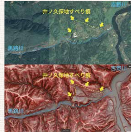
写真2: 国土地理院衛星画像図(上)と赤色立体図(下) 赤色立体図は赤いところほど傾斜がきつく、白いところほど緩やかな様子を表している。
