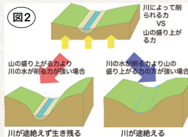
川が途絶えず生き残る場合と川が途絶えてしまう場合。四国山地を北流する吉野川などは川の水の削る力が強かった。
