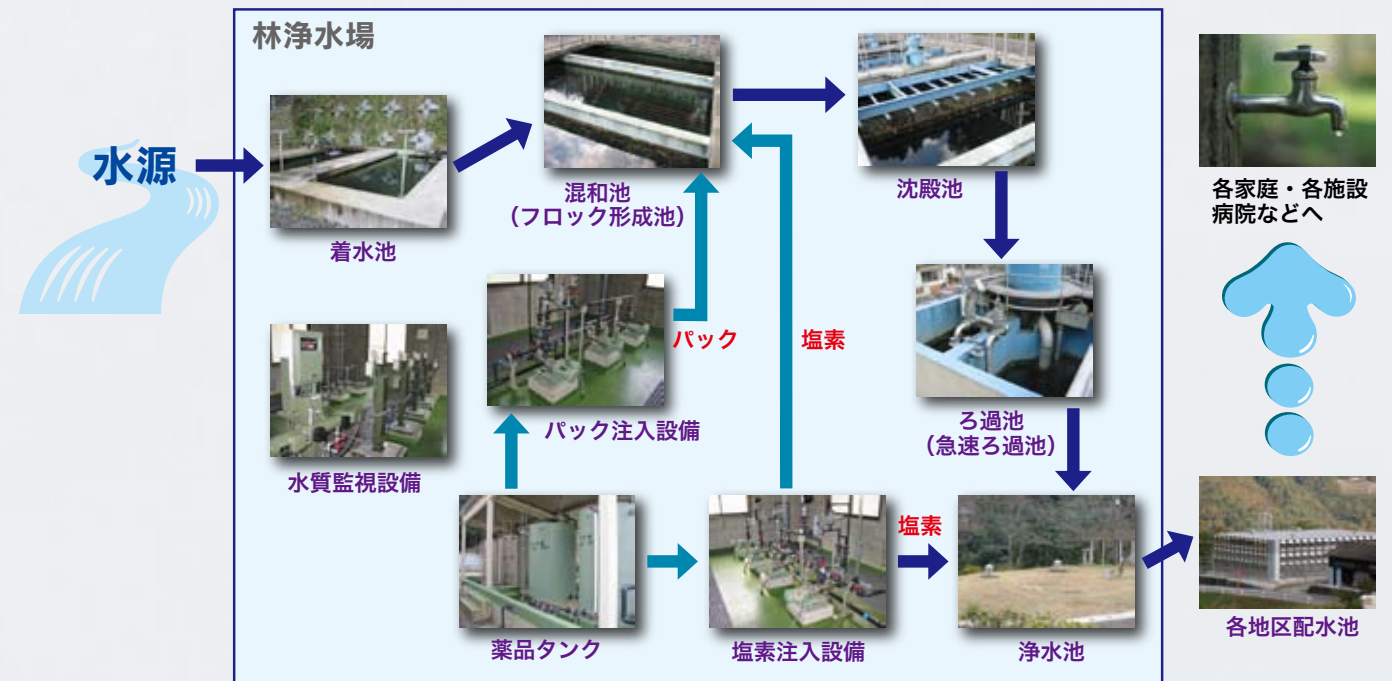
■水道水ができるまで(上水道の例) ※地区によって方式は異なります
