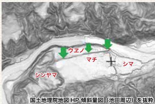
【図1】池田市街地の傾斜量図。緑の矢印部分が中央構造線（池田断層）の断層崖
